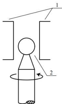
图 5 可换球测头直径偏差测量示意图
