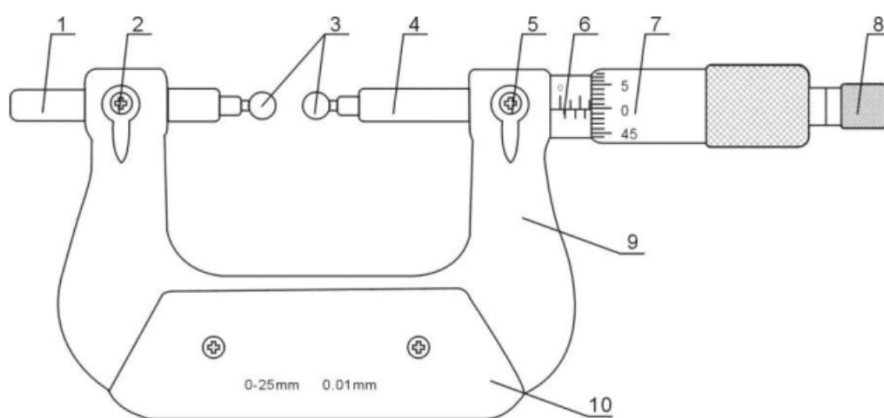
图 1 齿轮千分尺
